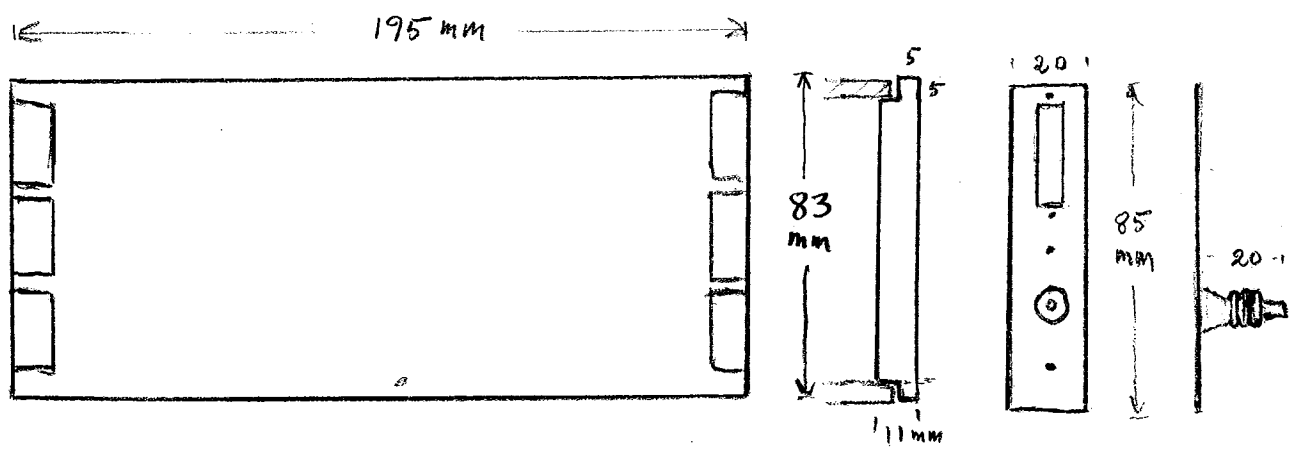
Innerlådan
