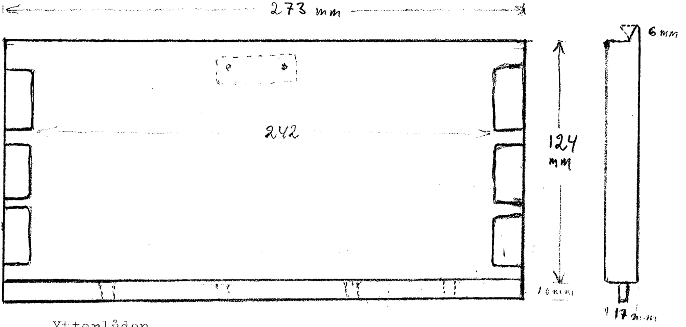
Ytterlådan
